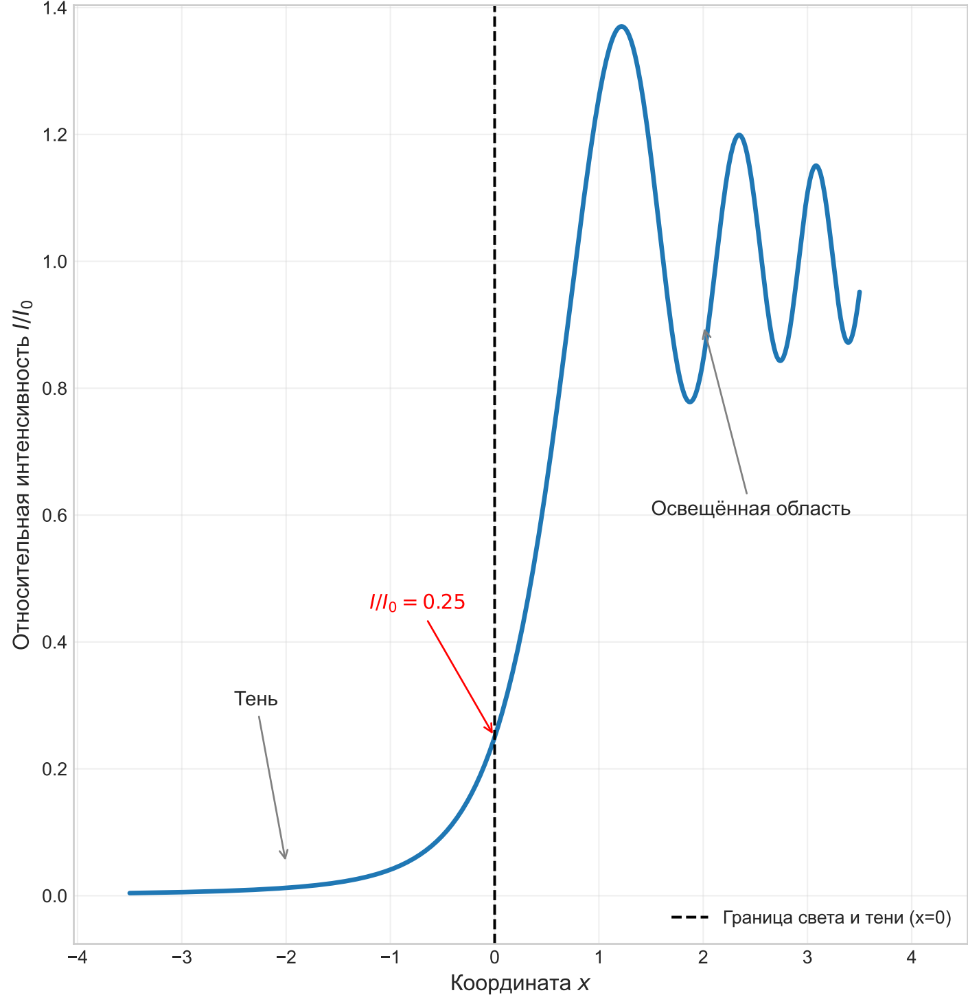
Распределение интенсивности на границе света и тени
