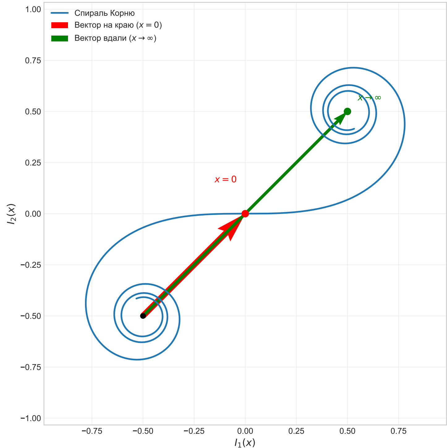
Спираль Корню и векторы амплитуд
